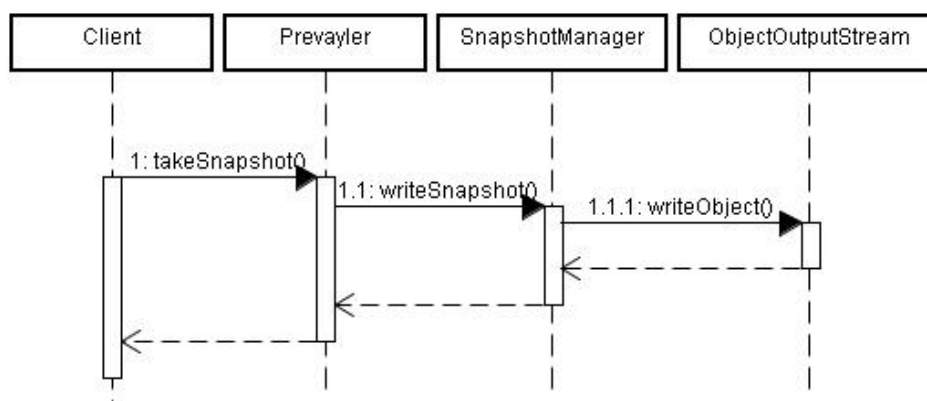
Figura 4. Persistência requisitada por um cliente do Prewayler.
