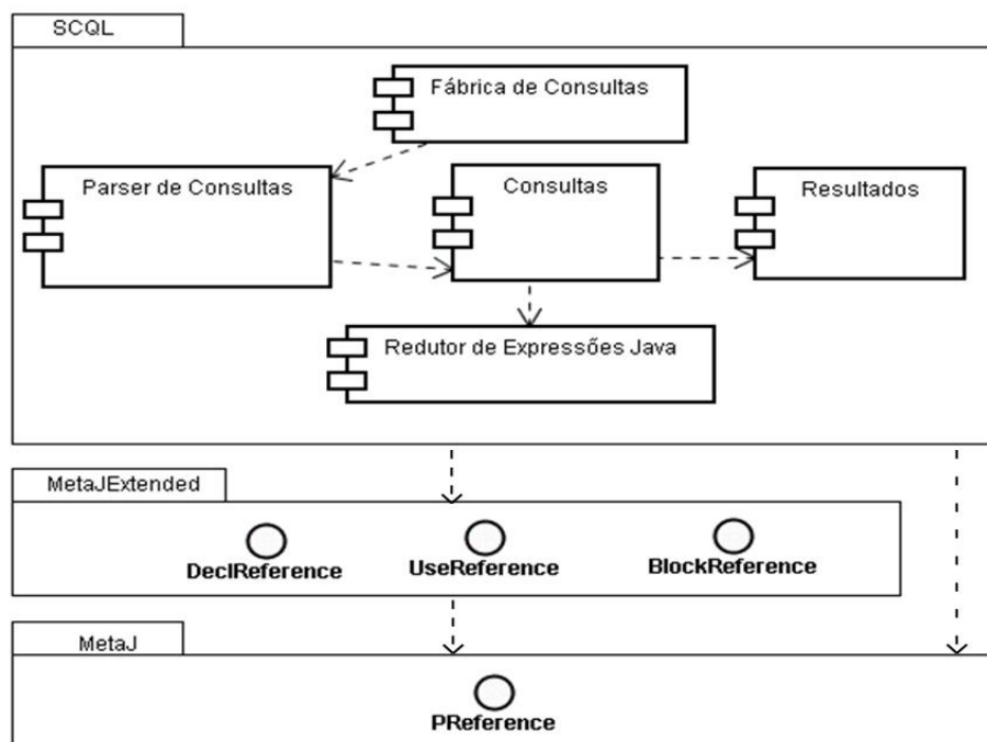
Figura 3. Arquitetura Geral de SCQL.
